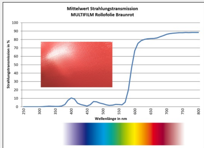
Foto 2: Der spezielle Rot-Ton der Folie öffnet im gewünschten Wellenlängenbereich
